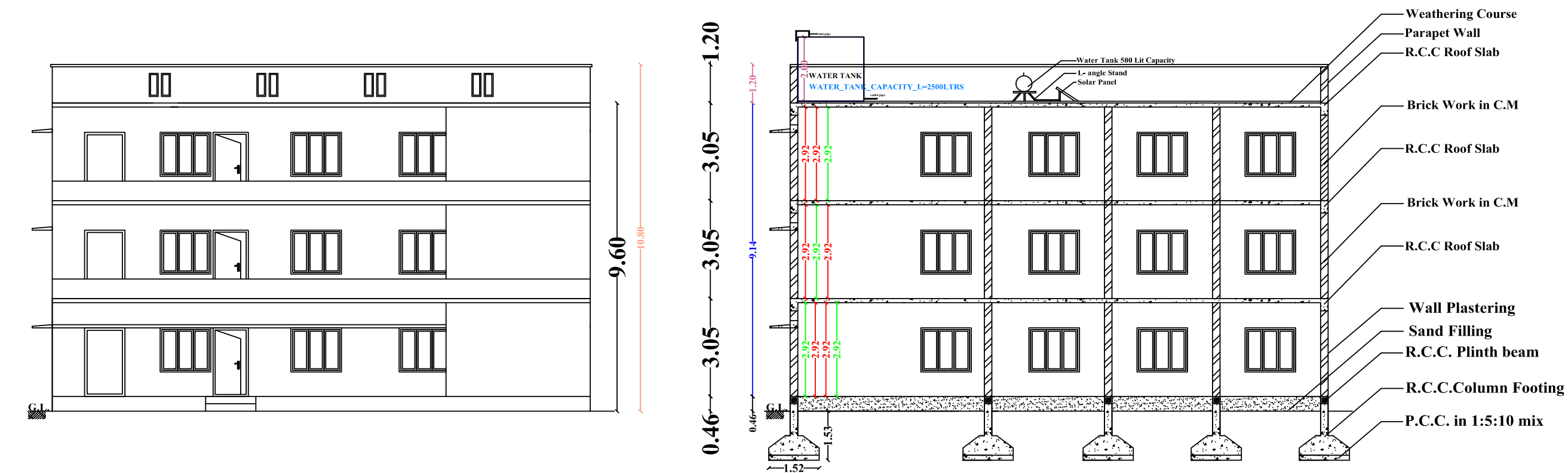
ELEVATION
