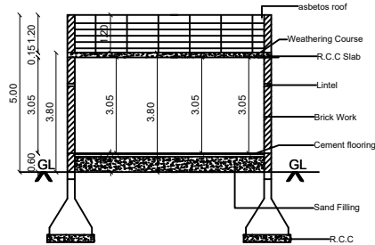
SECTION ON'AB'
