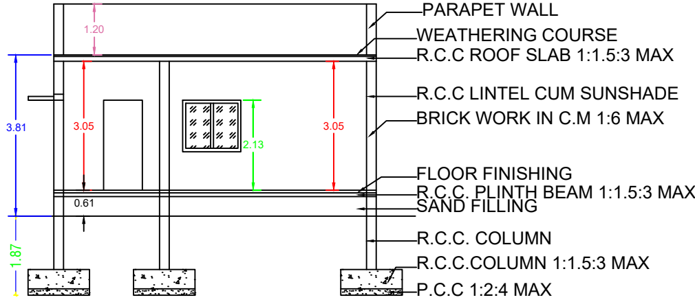
SECTION - AB
