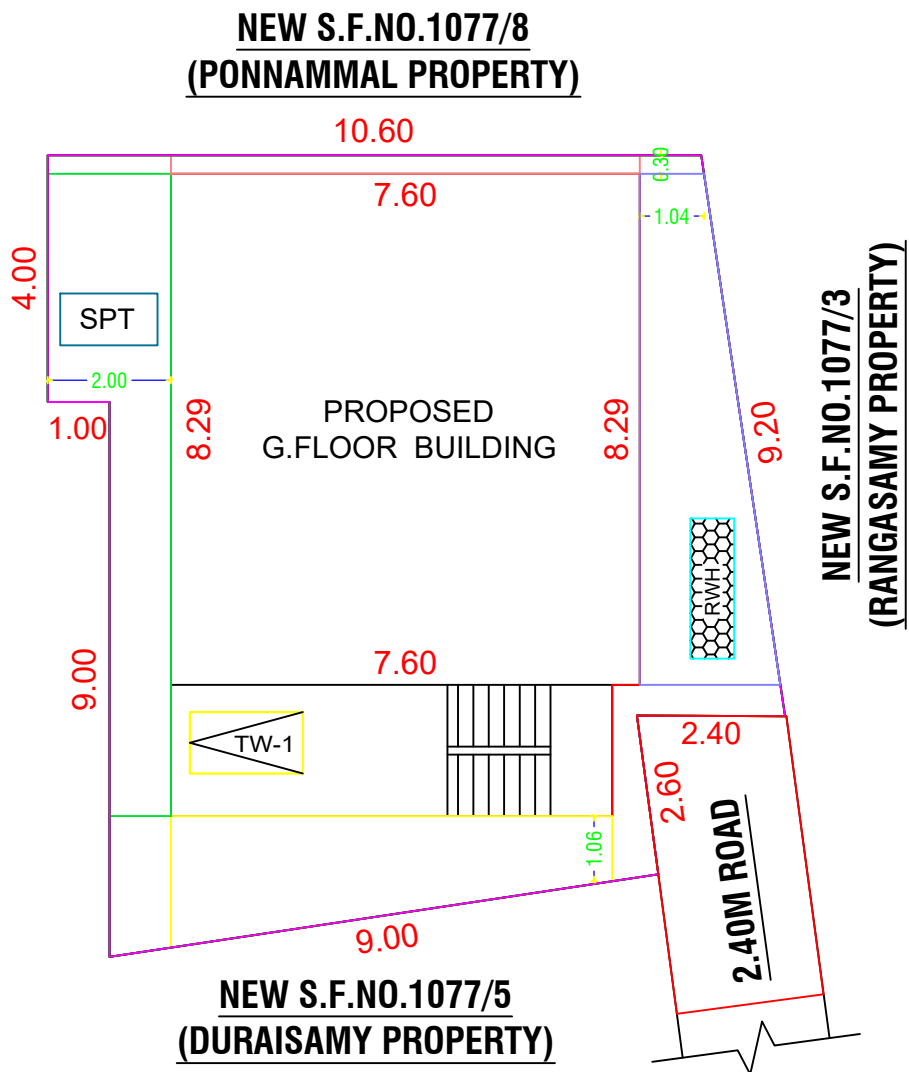
SITE PLAN 1:100
