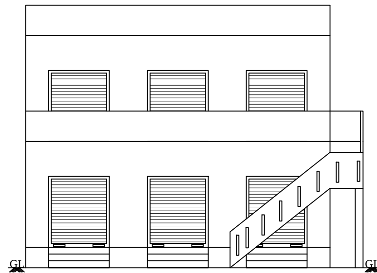
ELEVATION
