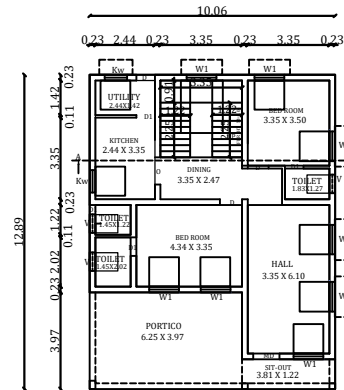
PRO. G. FLOOR PLAN
