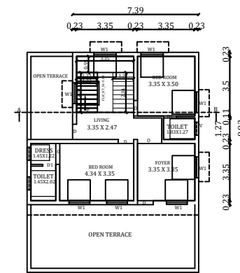
PRO. F. FLOOR PLAN
