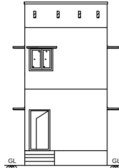
ELEVATION
