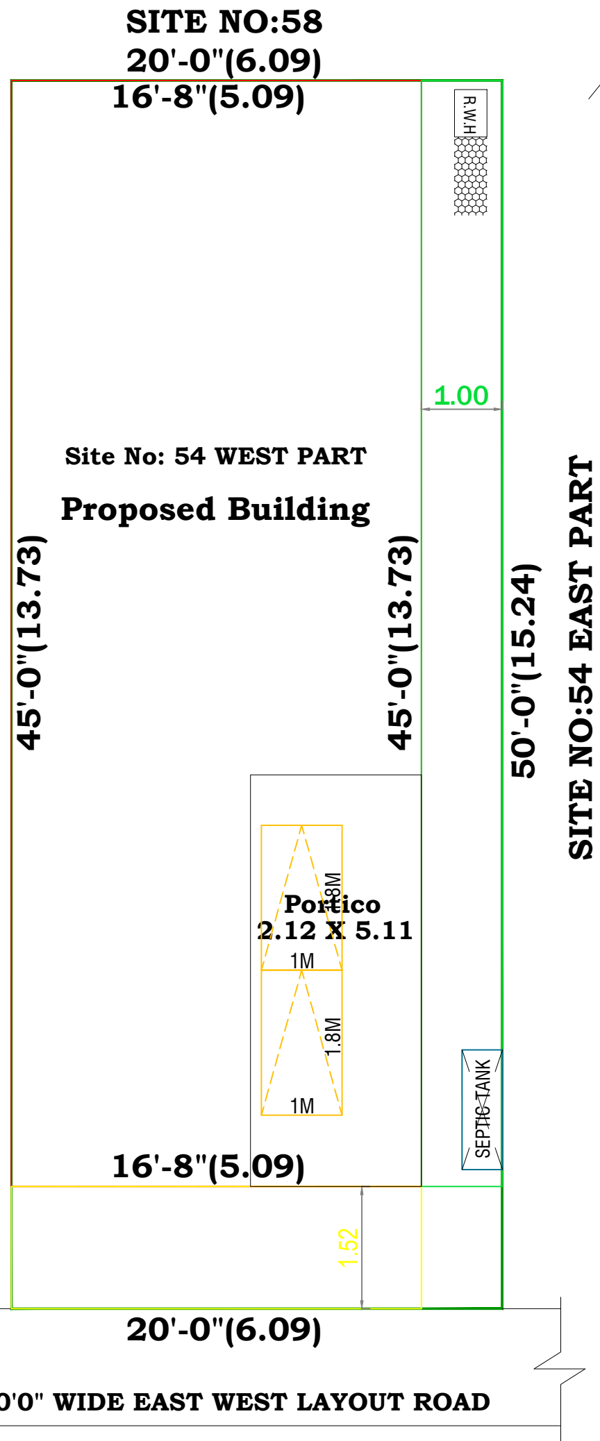
SITEPLAN
