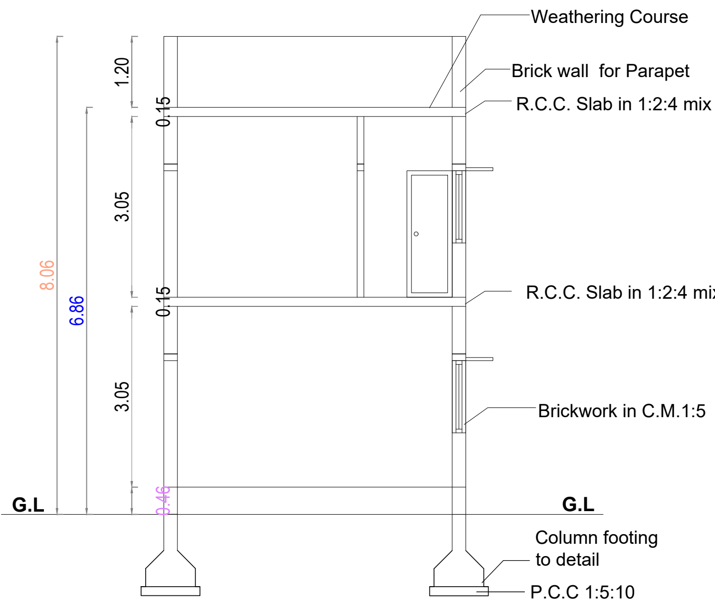
SECTION A-A
