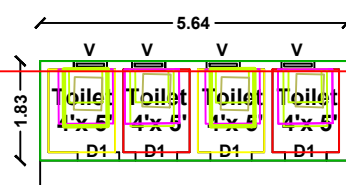
Toilet Plan
