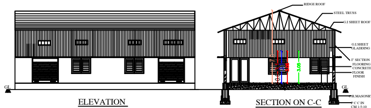
ELEVATION
