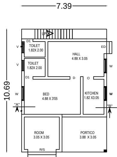
PRO. G.F PLAN
