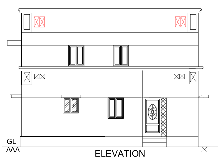
ELEVATION
