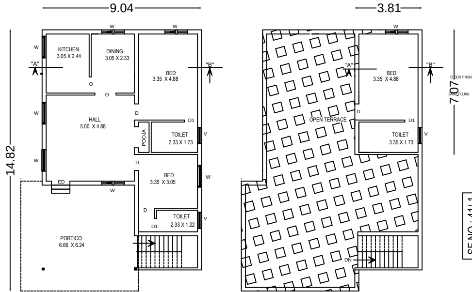
PRO. G.F. PLAN
