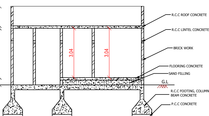
SECTION - A-B
