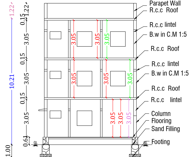
SECTION A-B
