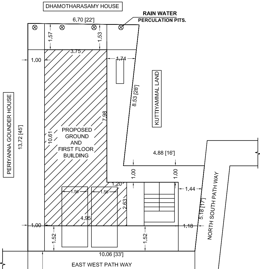
ITE PLAN
