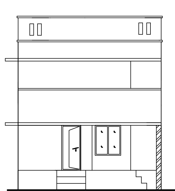
ELEVATION
