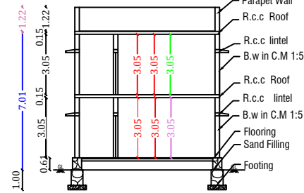
SECTION A-B
