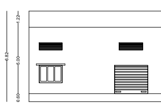
ELEVATION
