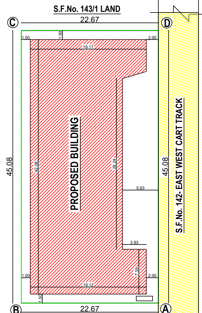
S.F.No. 143/1 LAND SITE PLAN
