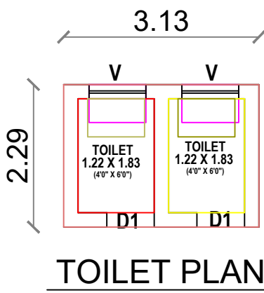
TOILET PLAN
