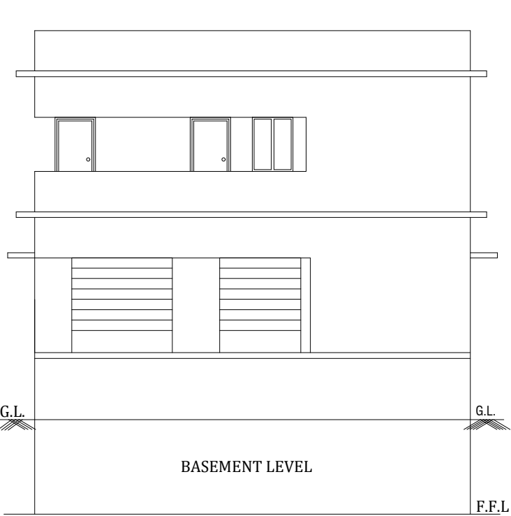
ELEVATION
