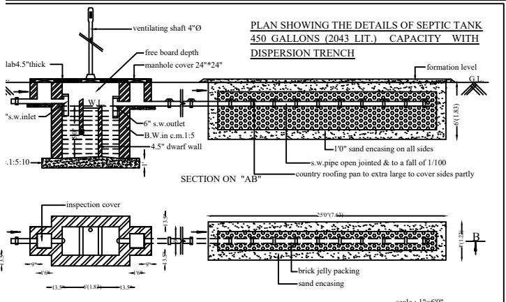
LAN
