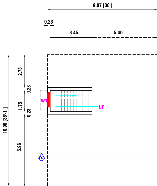
LAN
