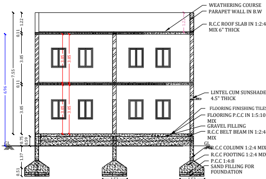
SECTION A-B
