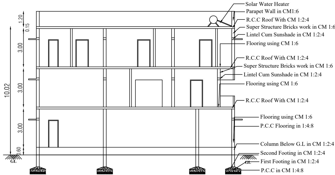
SECTION A-B
