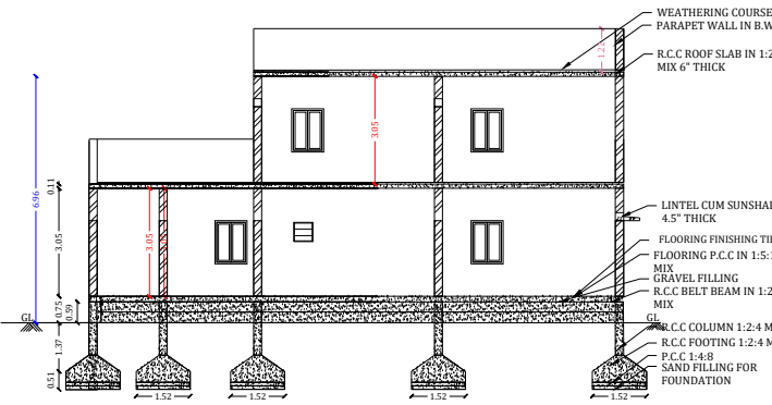
SECTION A-B
