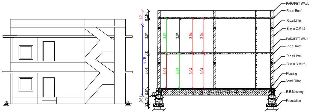
ELEVATION
