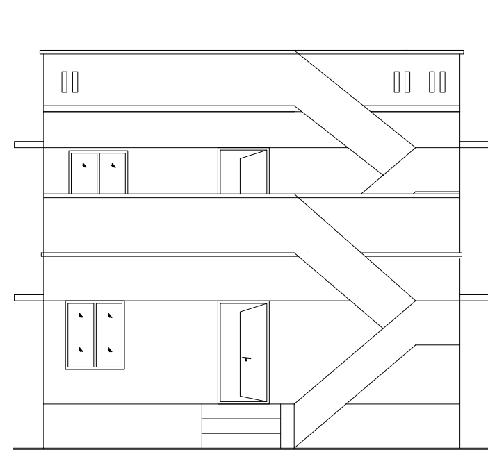
ELEVATION
