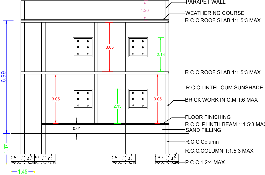
SECTION - AB
