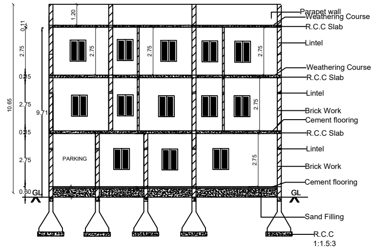
SECTION A-B
