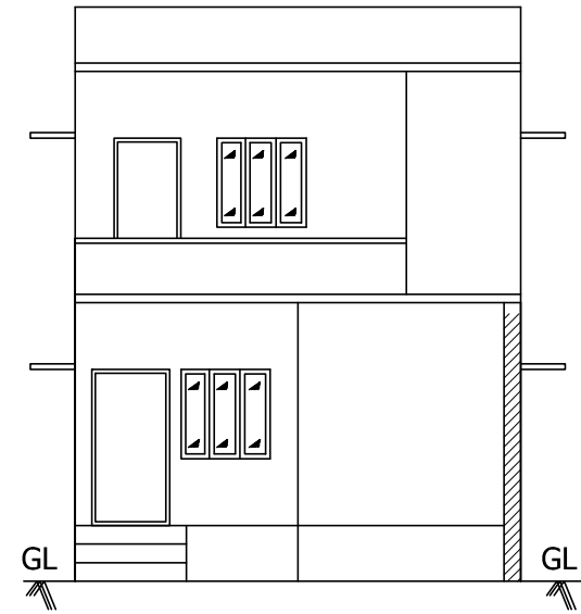
ELEVATION
