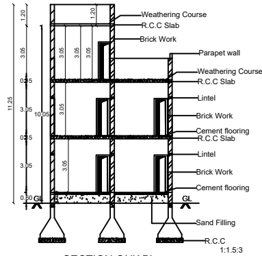
SECTION ON'AB'
