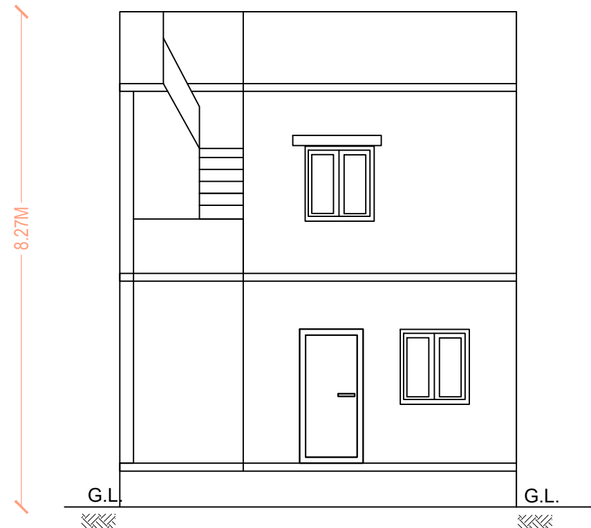
ELEVATION
