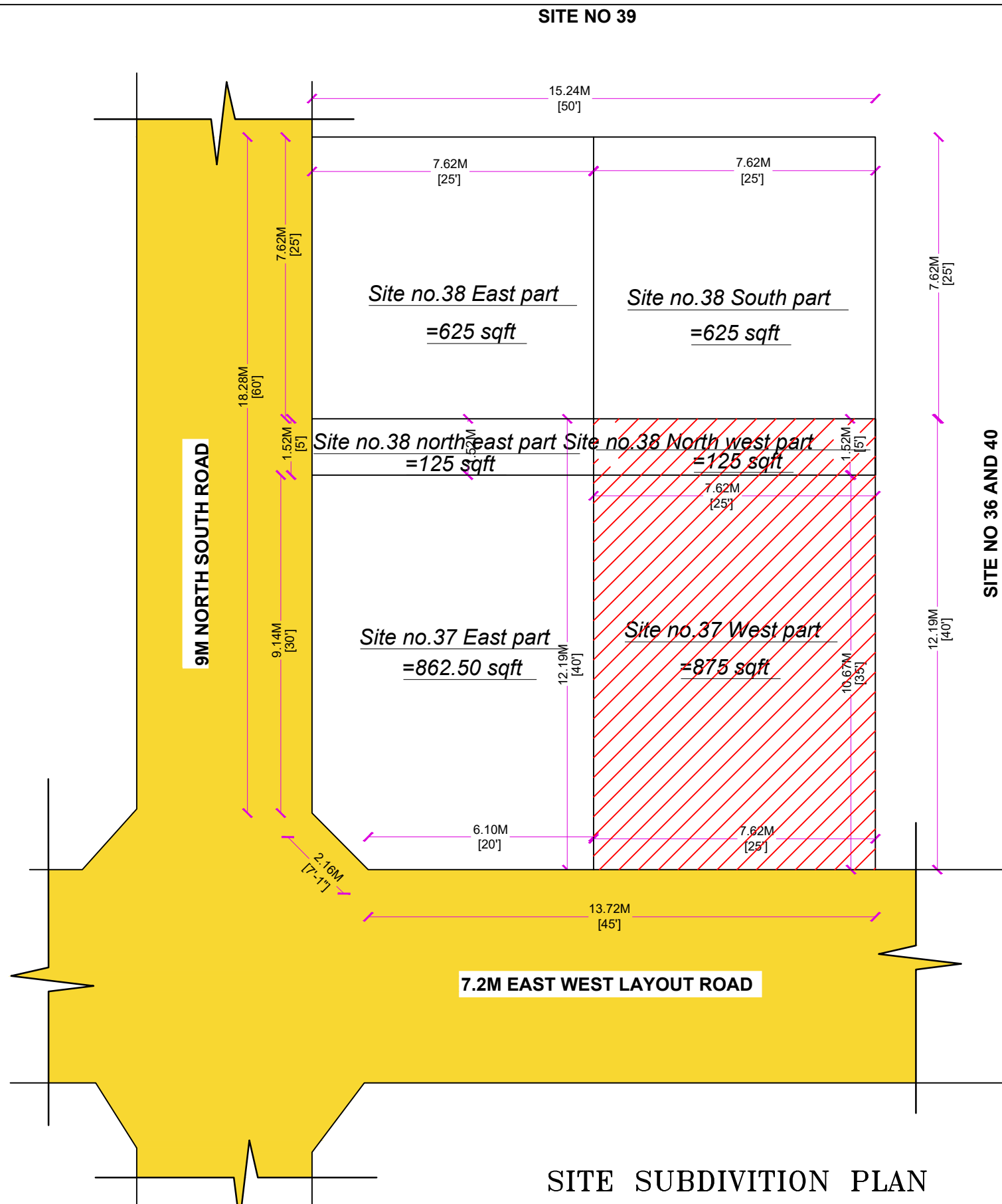
SITE SUBDIVISION PLAN
