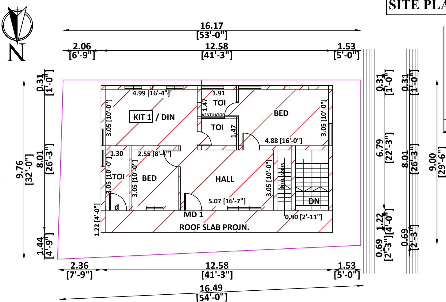
PRO. FIRSTFLOOR PLAN -1 RESI. UNITS
