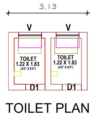
TOILET PLAN
