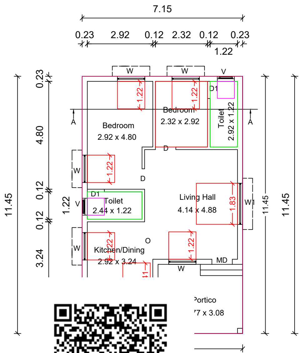
DOOR PLAN
