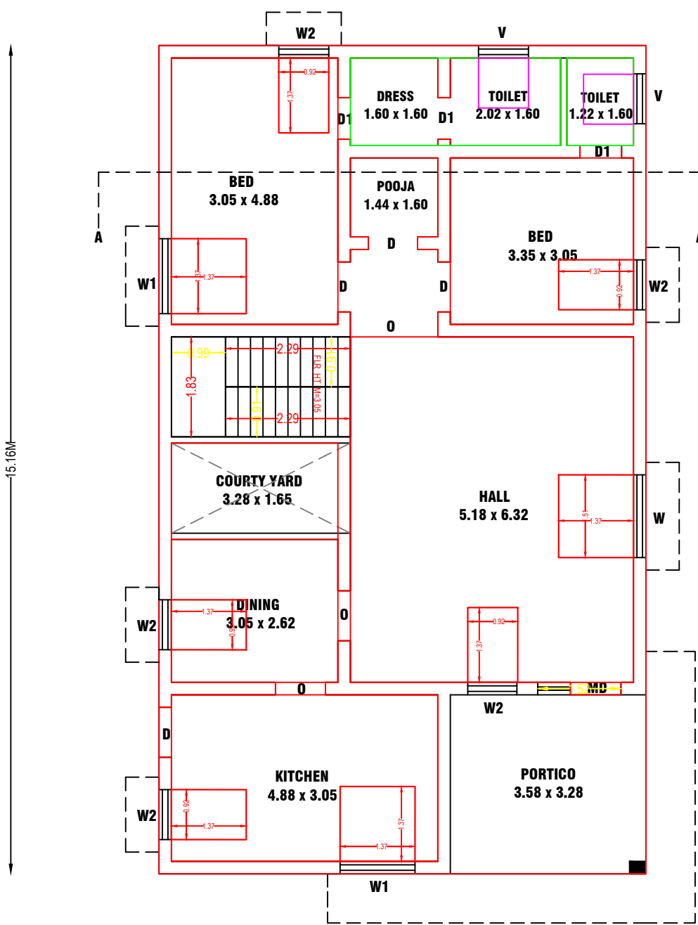
FLOOR PLAN E1:100
