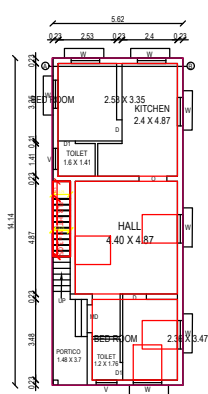
EXISTING FLOOR D.NO:3
