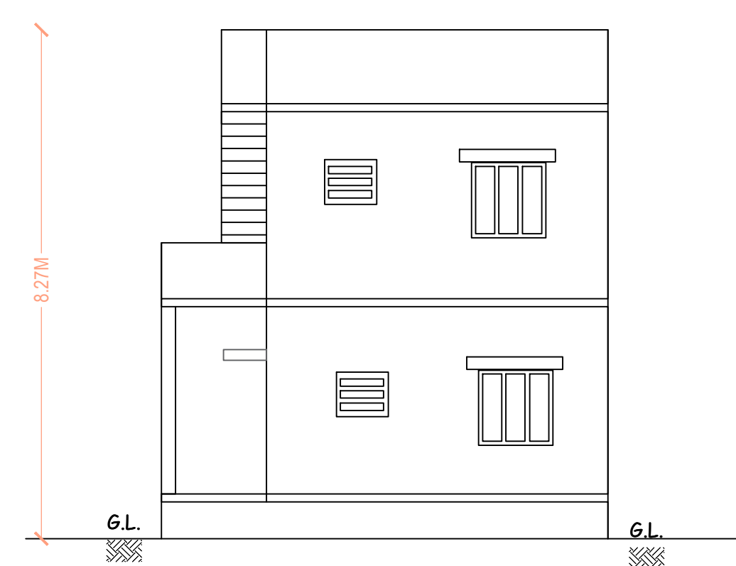
ELEVATION
