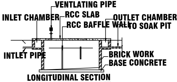
LONGITUDINAL SECTION
