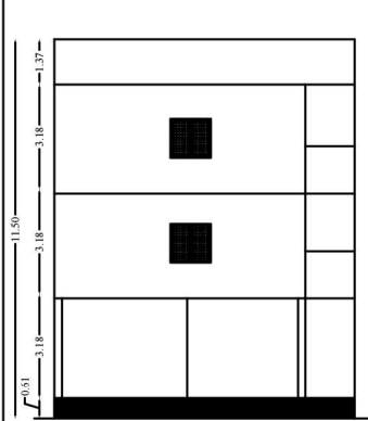
ELEVATION
