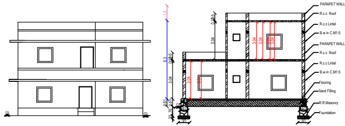
ELEVATION
