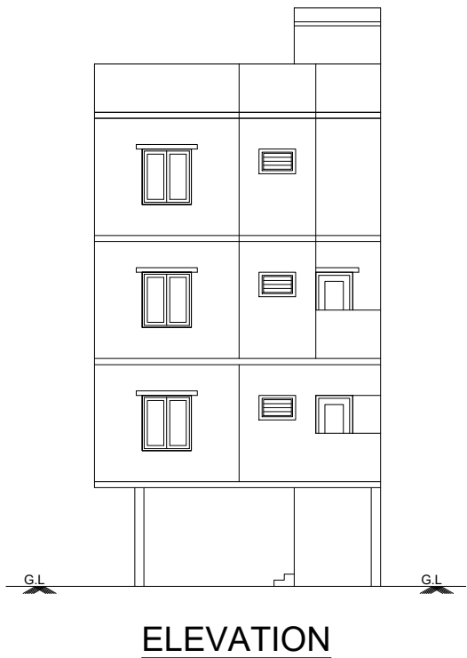
ELEVATION
