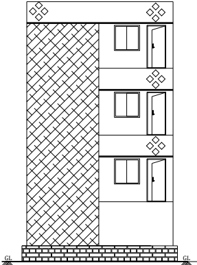
ELEVATION
