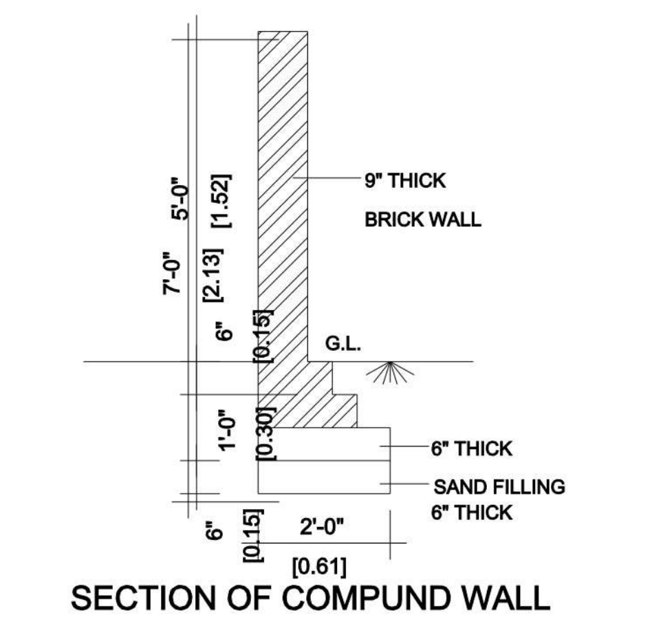
SECTION OF COMPUED WALL
