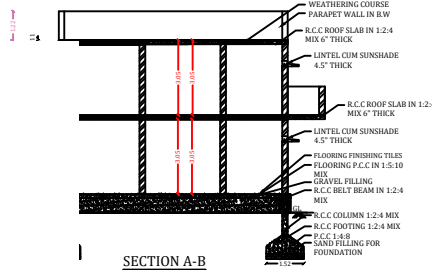
SECTION A-B
