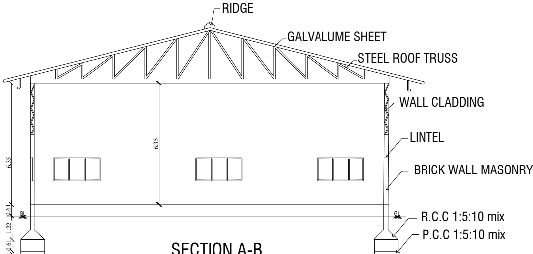
SECTION A-B
