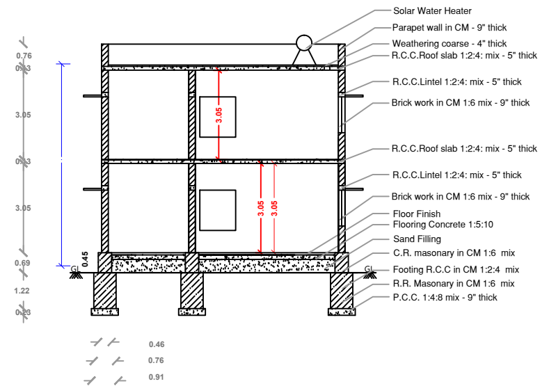
SECTION 'AB'
