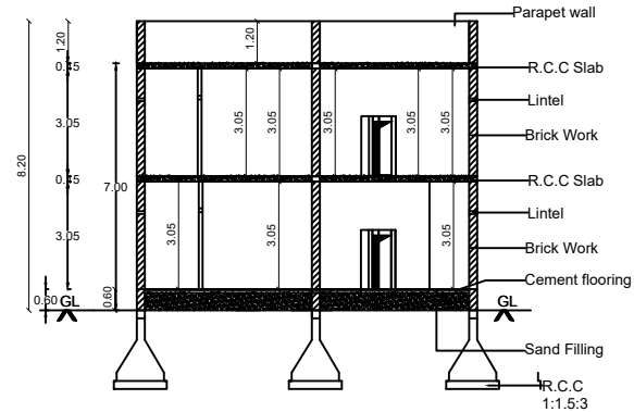
SECTION ON'AB'
