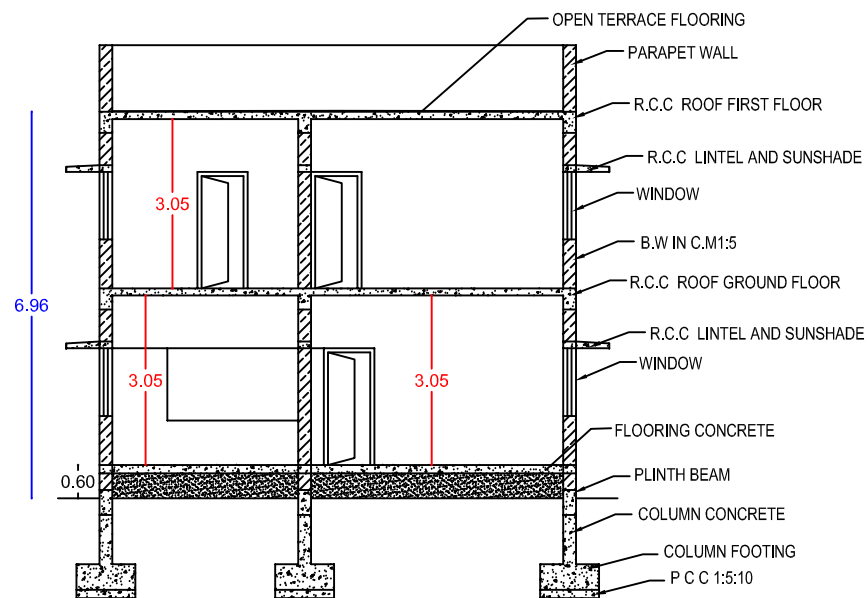
SECTION - AB
