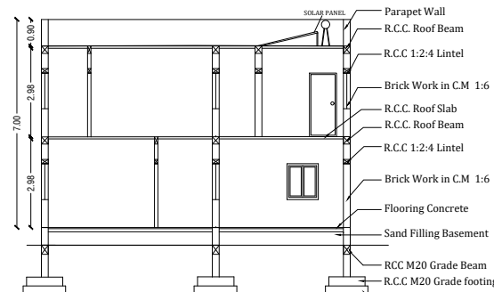
SECTION A-B
